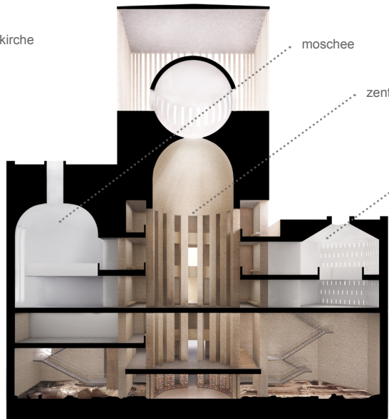
längsschnitt
