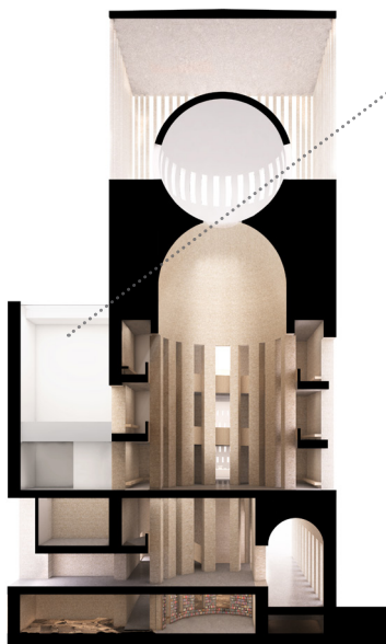
querschnitt
