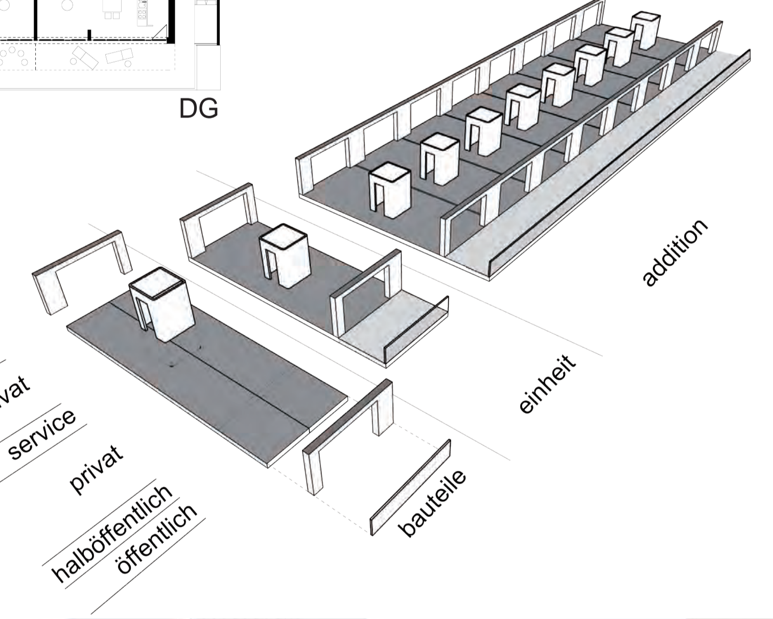
Pläne: Links: EG/1.OG/DG/Schnitt/1:250, Rechts: Aspern/Baufeld D13, Unten rechts: Wohnmodule Renderings: Ganz oben: Südsicht, Links: Nordansicht, Fotos: Unten links: Nordfassade, Mitte: Zugang Westseite Unten mitte: Südfassade Unten rechts: Nebengebäude für Gemeinschaftsräume und Atelier
