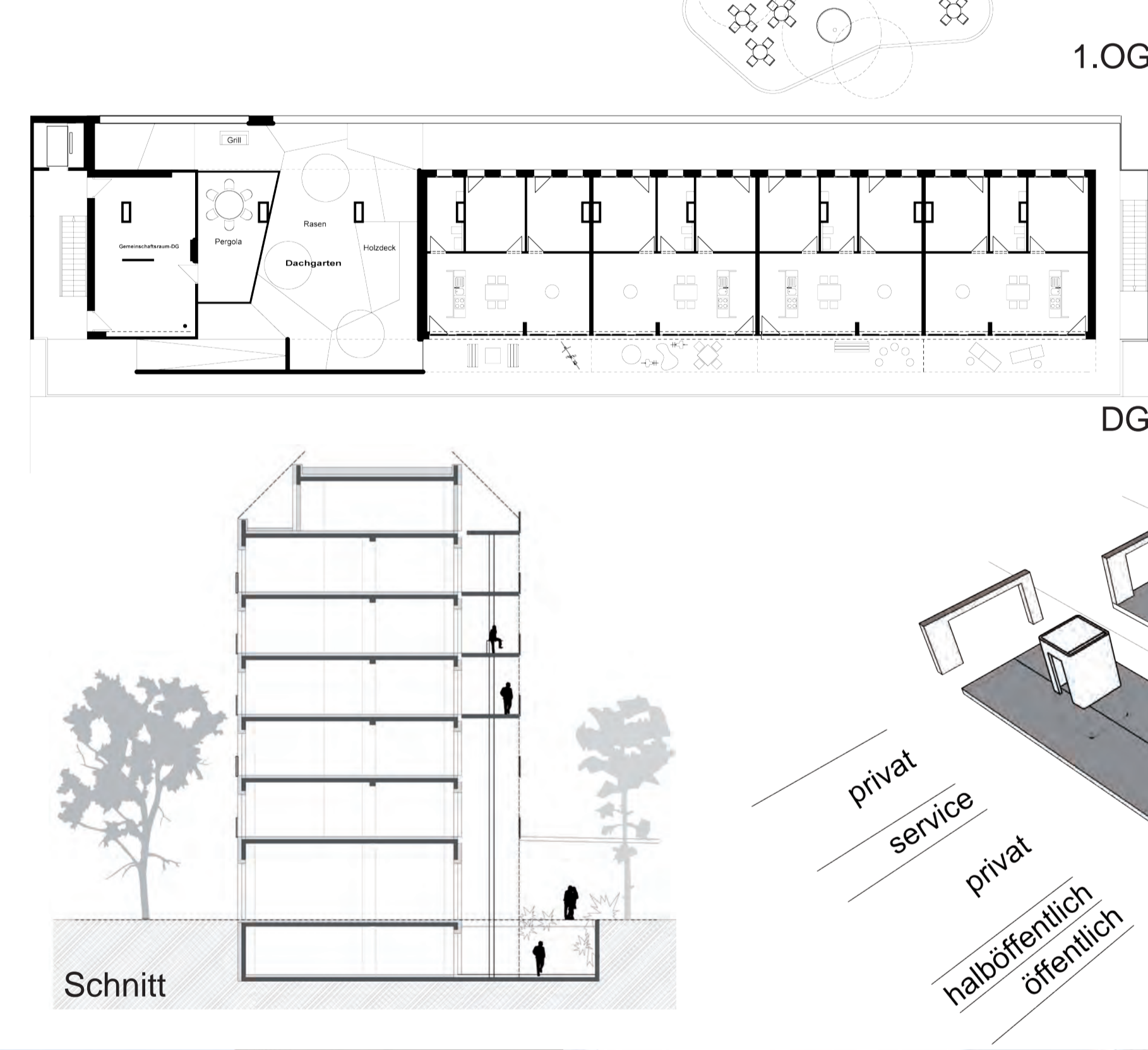
Pläne: Links: EG/1.OG/DG/Schnitt/1:250, Rechts: Aspern/Baufeld D13, Unten rechts: Wohnmodule Renderings: Ganz oben: Südsicht, Links: Nordansicht, Fotos: Unten links: Nordfassade, Mitte: Zugang Westseite Unten mitte: Südfassade Unten rechts: Nebengebäude für Gemeinschaftsräume und Atelier
