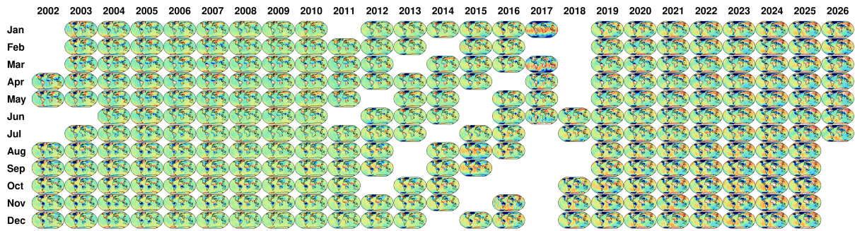
Abbildung 2: ITSG-Grace operational: Monatliche Massenänderungen
